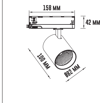
Mått/Dimension
