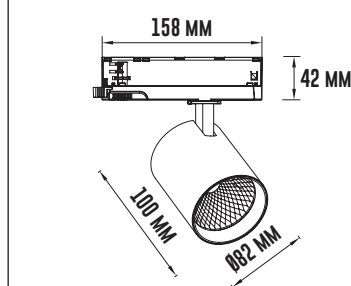
Mått/Dimension
